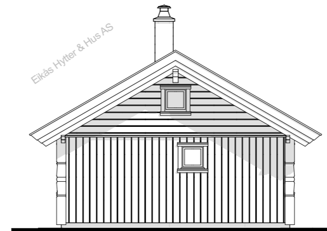
Fasade mot Øst
