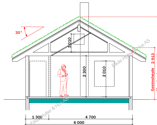
Snitt
