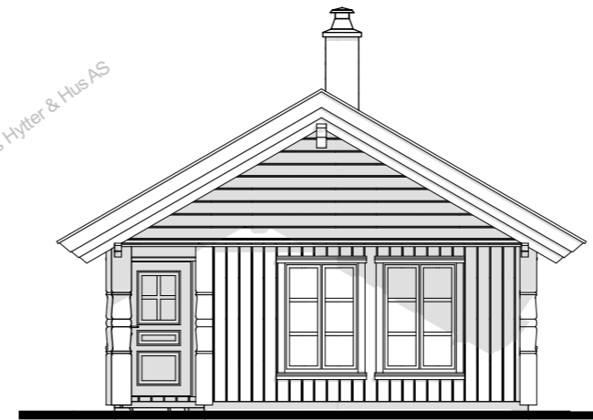
Fasade mot Vest
