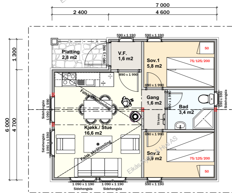
Hovedplan
