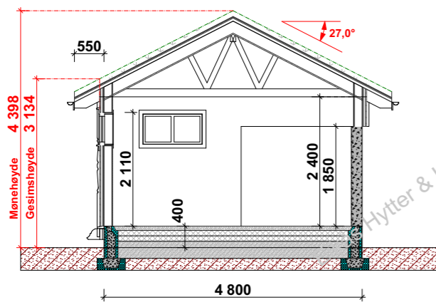
Snitt A-A
