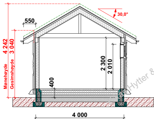
Snitt B-B
