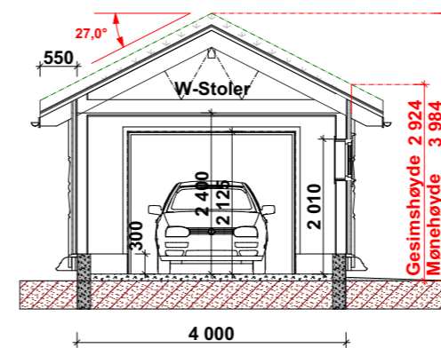
Snitt A-A
